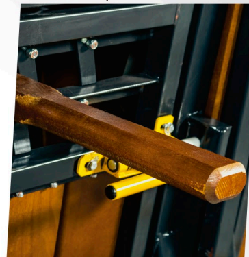
Cambão protetor de coice
