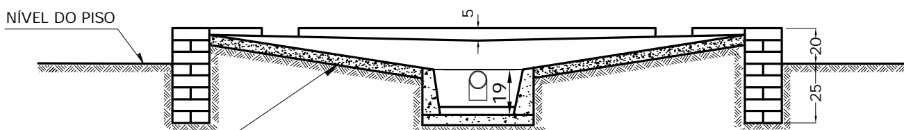
CORTE LONGITUDINAL
