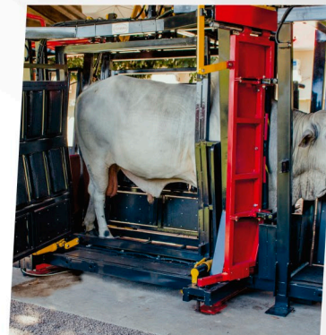
Portão lateral salva vidas
